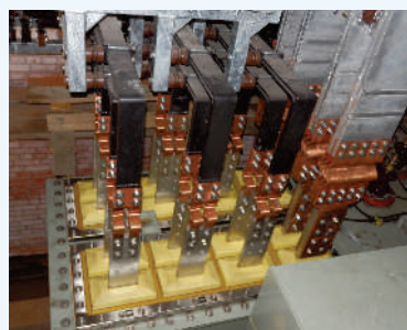
Wysokoprądowe systemy szynowe Przesył prądów do 200kA. Przemysł chemiczny i metalurgiczny.
